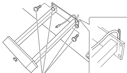
Parafusos de fixação de 6 x 20 mm
