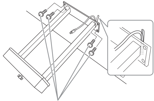
Parafusos de fixação de 6 x 20 mm
