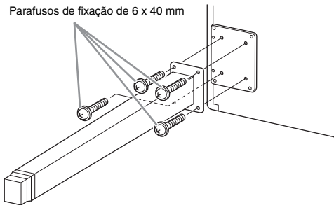
Parafusos de fixação de 6 x 40 mm
